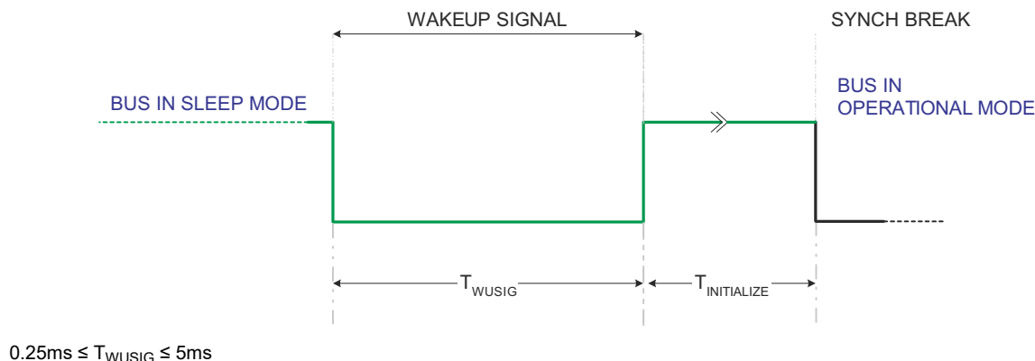
Figure 29-9. LIN Wakeup
