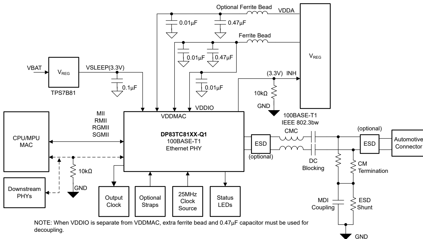
图 9-9. 带外设的典型 TC-10 应用
