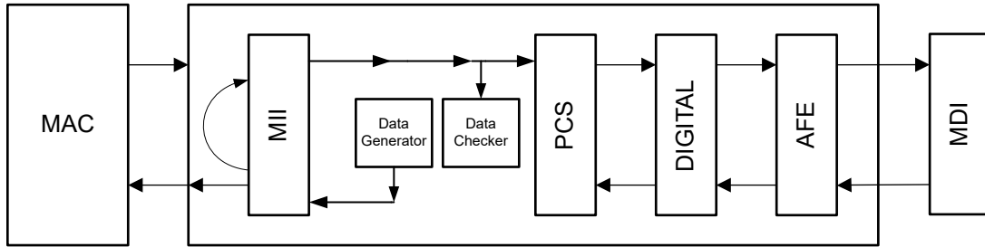
图 7-9. 带数据生成器的反向环回
