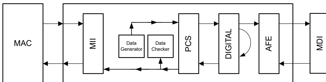
图 7-5. 带数据生成器的数字环回
