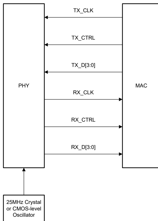
图 7-16. RGMII 连接
