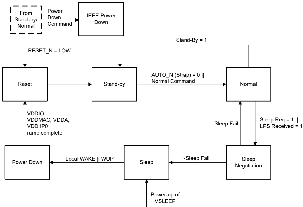
图 7-11. 功耗状态图
