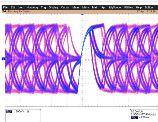
图 9-8. MDI 空闲流 (变量持久化)
