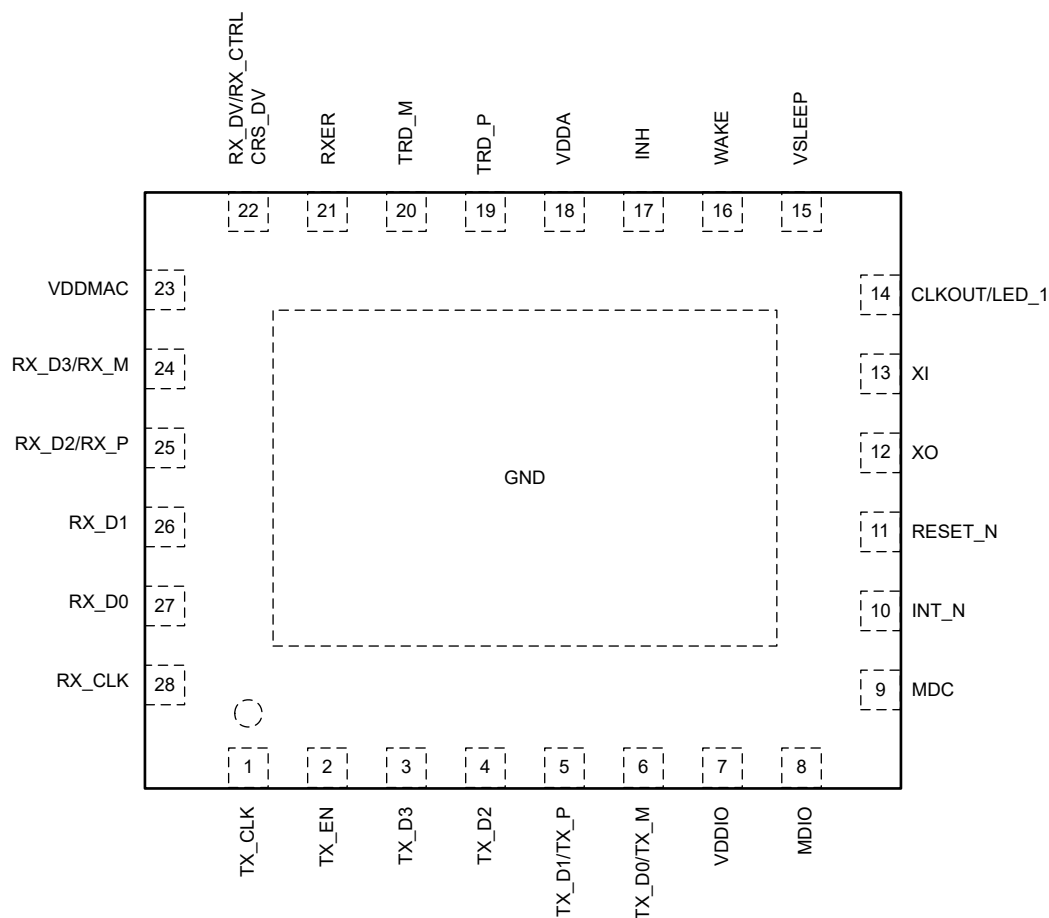
图 5-1. DP83TC813S-Q1 RHF 封装 28 引脚 VQFN 顶视图
