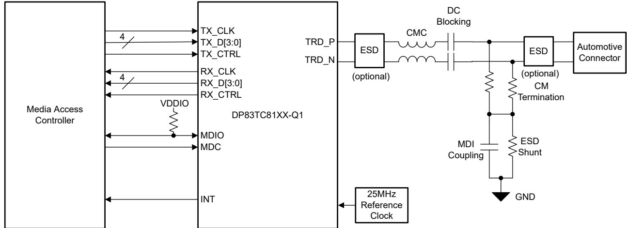
图 9-5. 典型应用 (RGMII)
