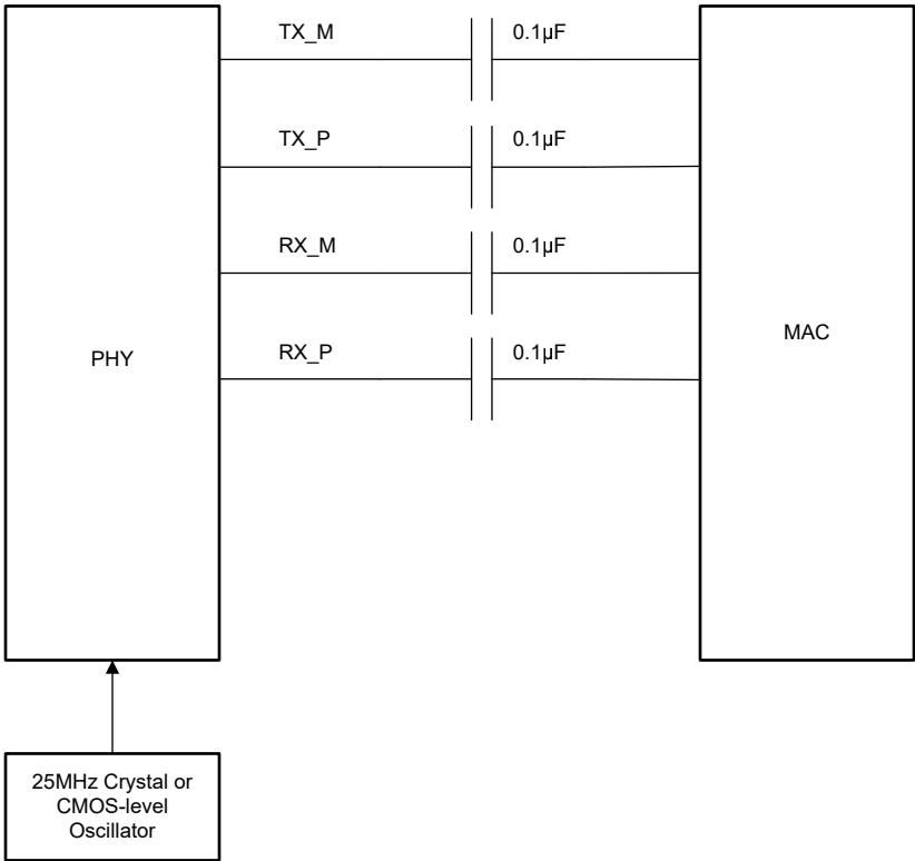
图 7-17. SGMII 连接
