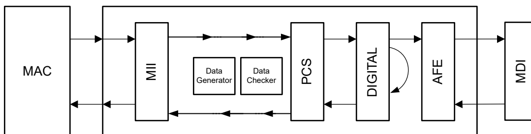
图 7-6. 不带数据生成器的数字环回
