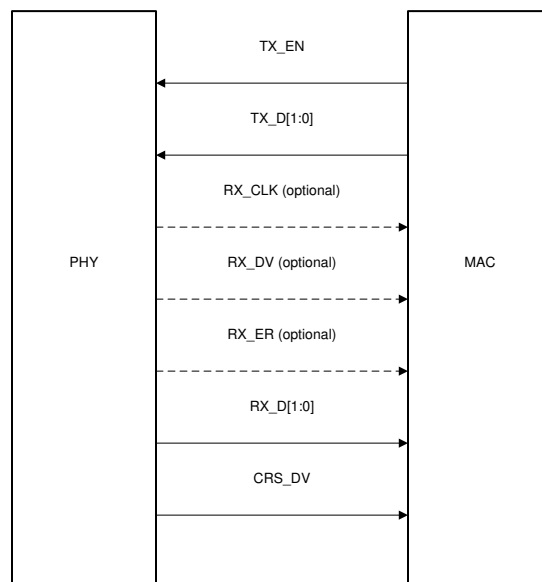
图 7-15. RMII 信号
