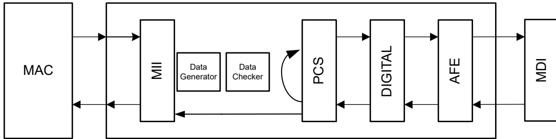
图 7-10. 不带数据生成器的反向环回
