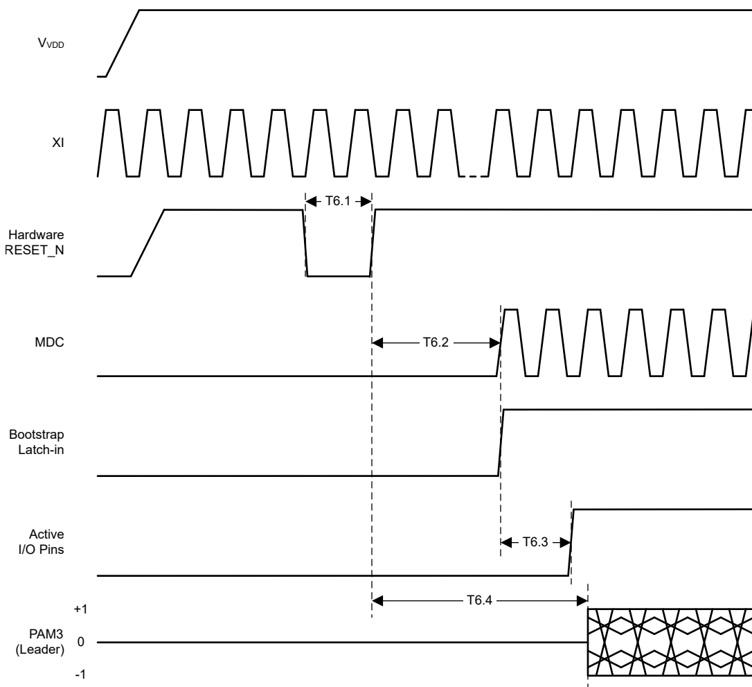
图 6-8. 复位时序
