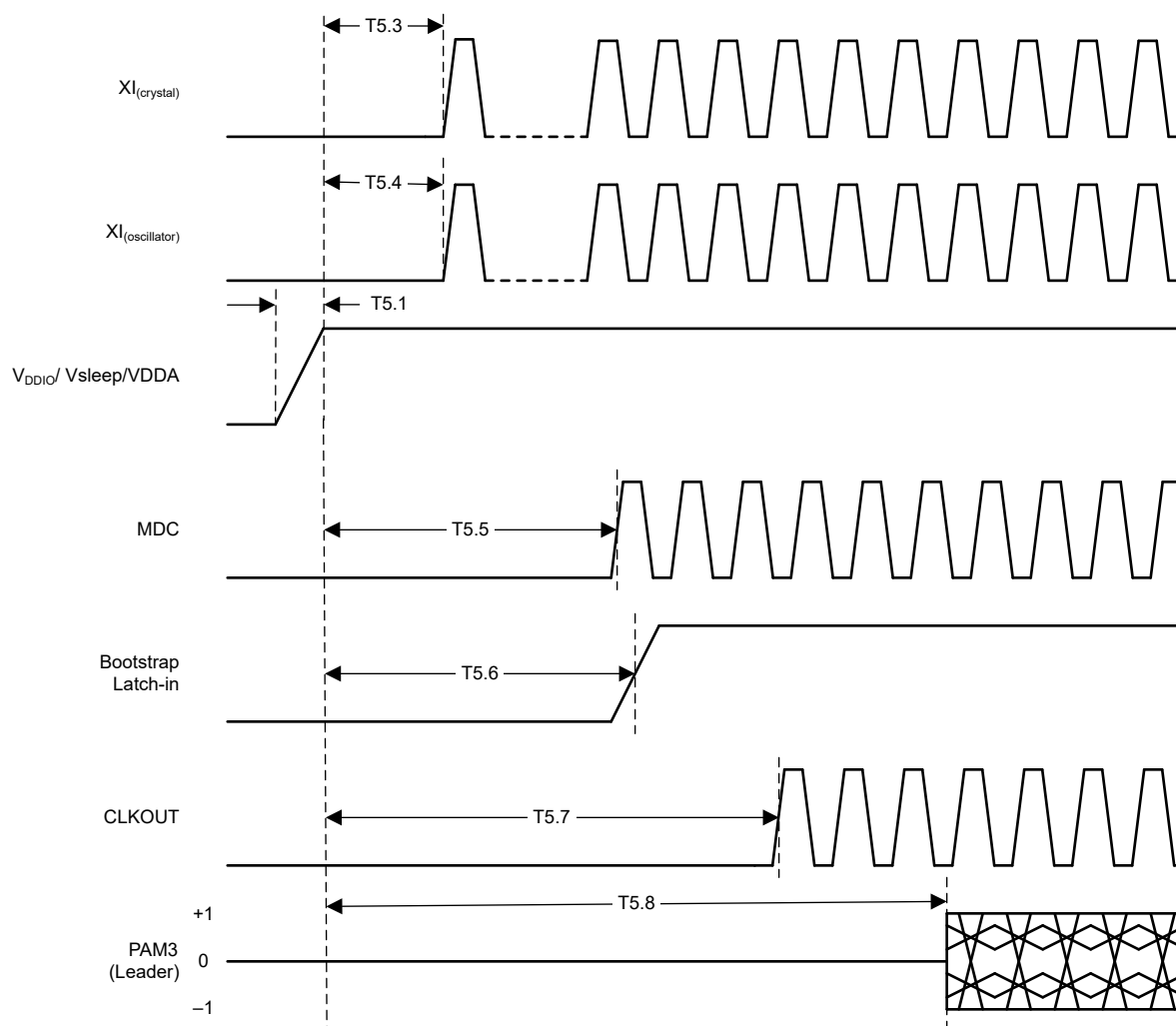
图 6-7. 上电时序
