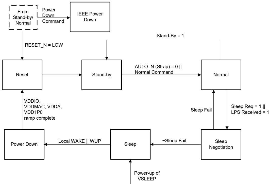
图 7-11. 功耗状态图
