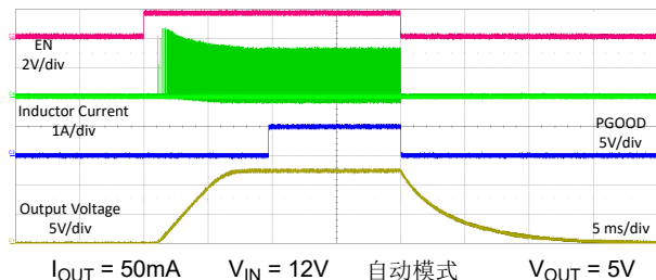
图 8-10. 启动
