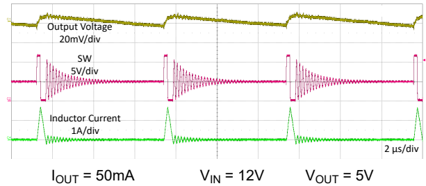
图 8-7. PFM 中的典型开关波形
