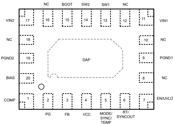
图 5-2. 20 引脚 RZT、WQFN-FCRLF 双相封装 (顶视图)
