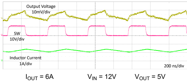
图 8-6. PWM 中的典型开关波形
