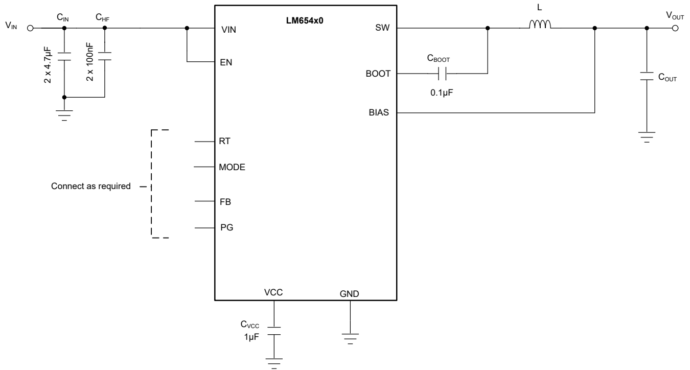
图 8-2. 采用 LM654X0-Q1 的固定输出电压模式示例应用电路
