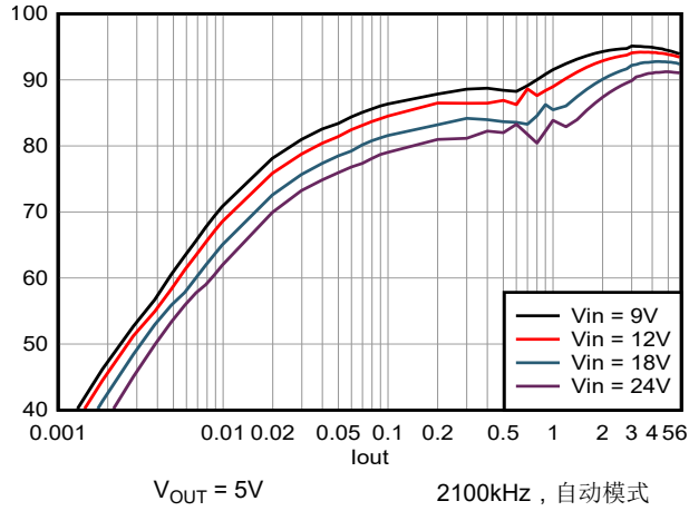
图 8-4. 效率
