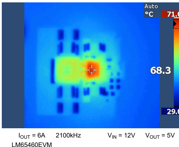
图 8-13. 热像图
