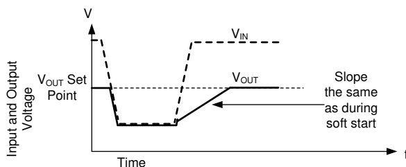
图 7-16. 输出电压下降时会缓慢恢复，以防止过冲和大浪涌电流
