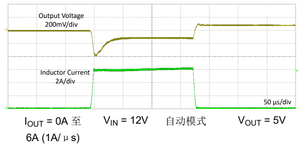
图 8-9. 负载瞬态 (AUTO)
