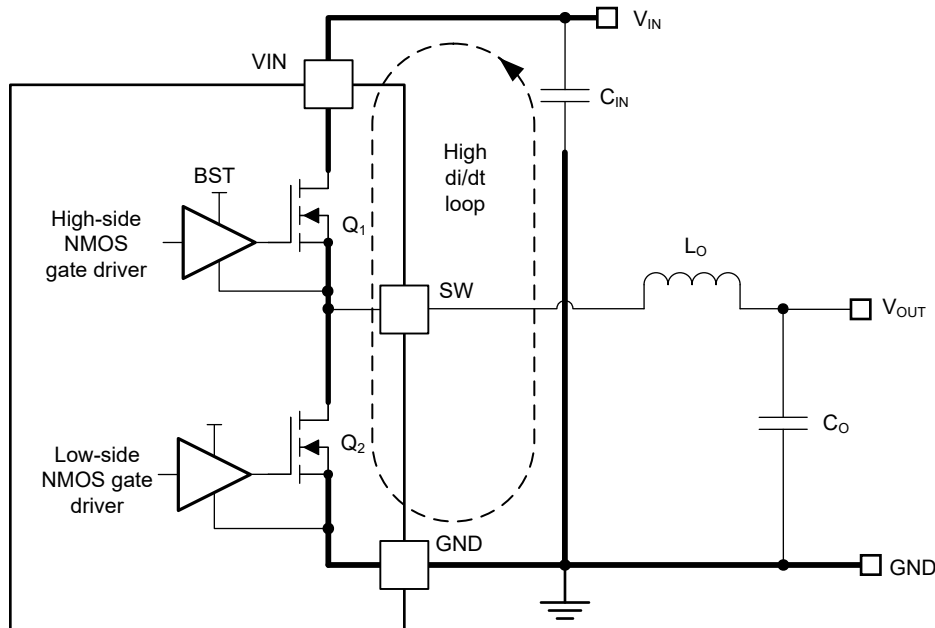
图 8-14. 具有快速边沿的电流环路
