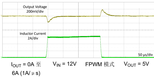
图 8-8. 负载瞬态 (FPWM)
