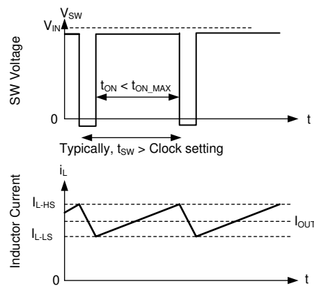
图 7-10. 电流限值波形
