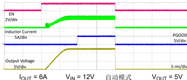
图 8-11. 启动
