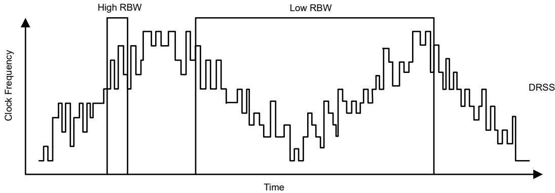
图 7-8. 双随机展频实现
