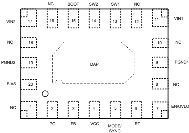
图 5-1. 20 引脚 RZT、WQFN-FCRLF 单相封装 (顶视图)
