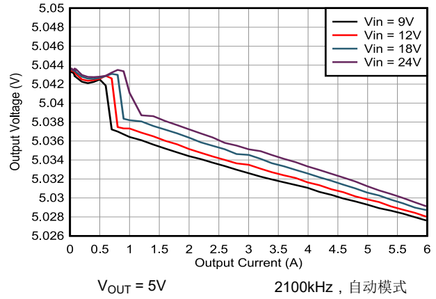
图 8-5. 线性 and 负载调整率
