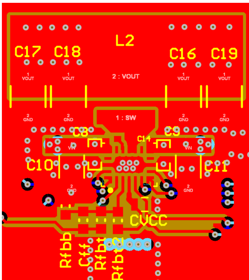
图 8-15. 布局示例
