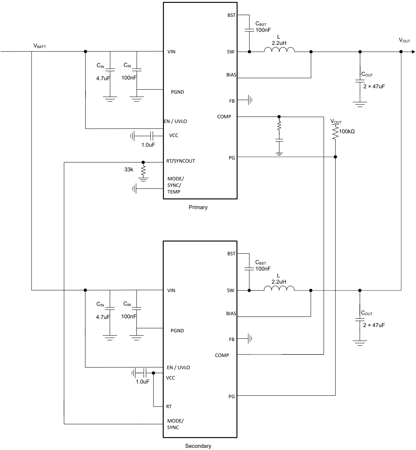
图 7-6. 典型固定 3.3V Vout 400kHz 双相原理图
