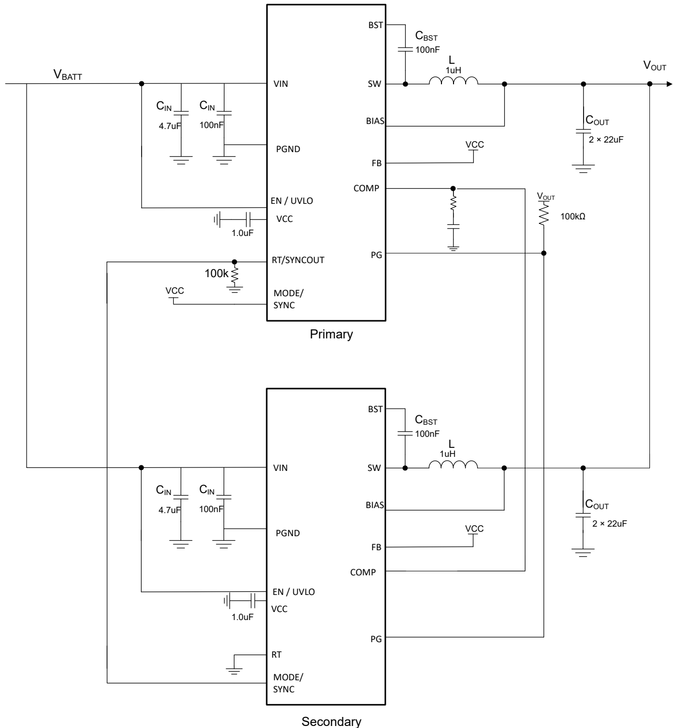
图 7-7. 典型固定 5V Vout 210kHz 双相原理图
