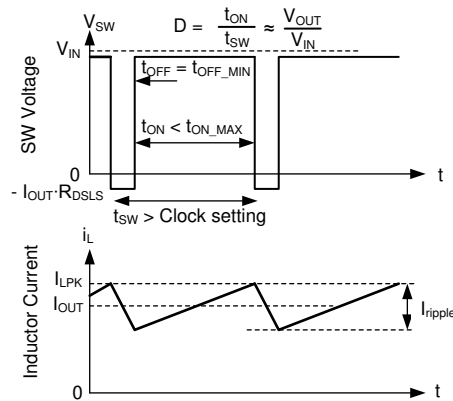
图 7-14. 压降中的频率和输出电压
