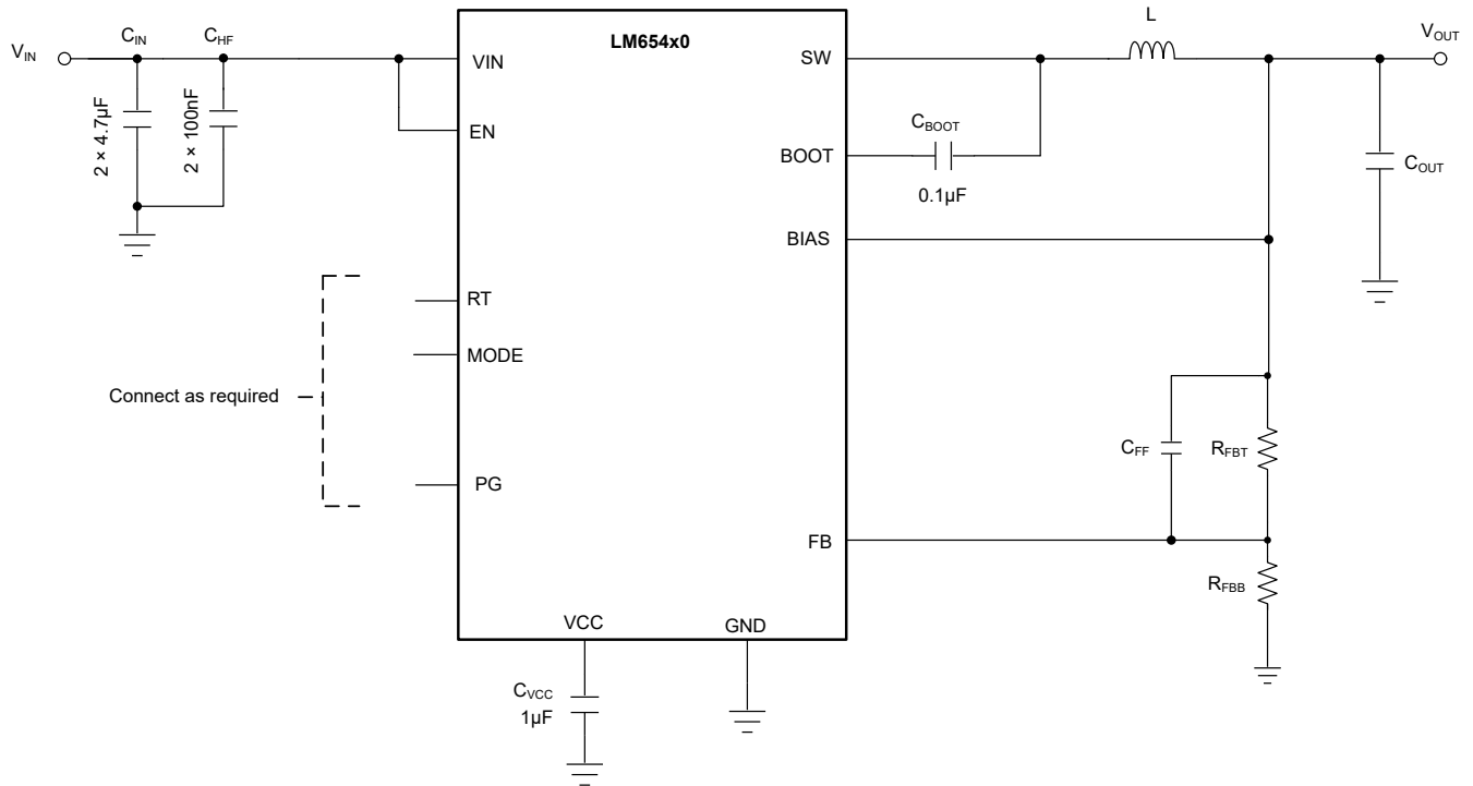
图 8-1. LM654x0-Q1 可调输出电压模式下的示例应用电路
