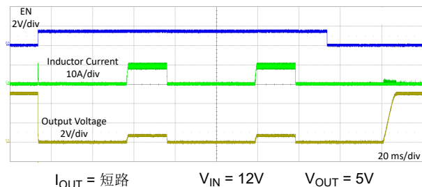
图 8-12. 短路
