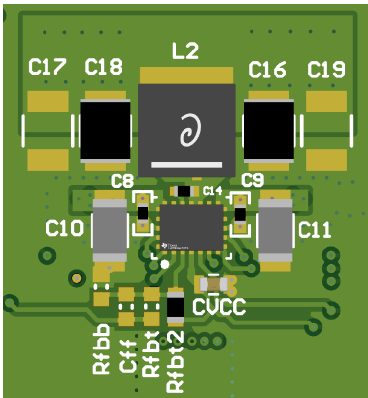
图 8-16. PCB 图像
