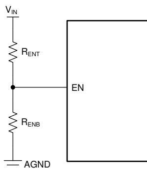
图 7-6. 外部 UVLO 应用的设置
