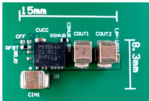
EVM 布局典型设计尺寸 – 15mm × 8.3mm
