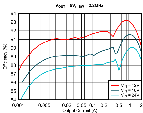
效率与输出电流之间的关系
