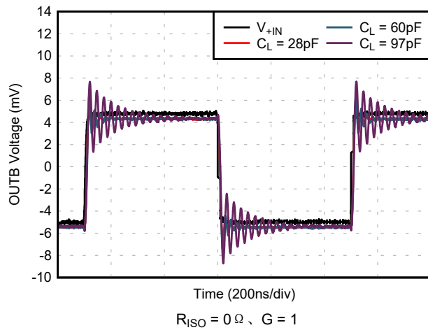
图 5-21. 辅助放大器微小信号阶跃响应
