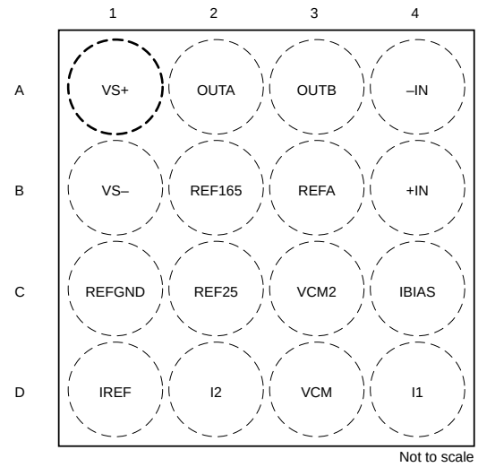
图 4-2. YBH 封装，16 引脚 DSBGA (俯视图)
