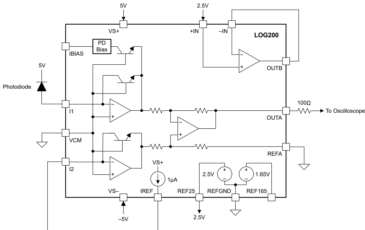
图 7-5. LOG200 光学电流检测应用
