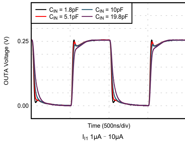
图 5-23. 不同 C_{\text{IN}} 的阶跃响应
