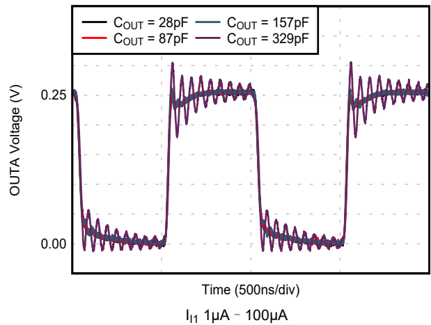
图 5-24. 不同 C_{\text{OUT}} 的阶跃响应
