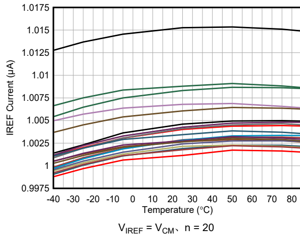
图 5-35. I_{REF} 与温度间的关系
