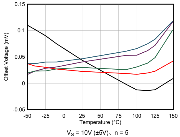
图 5-34. 辅助放大器偏移与温度间的关系
