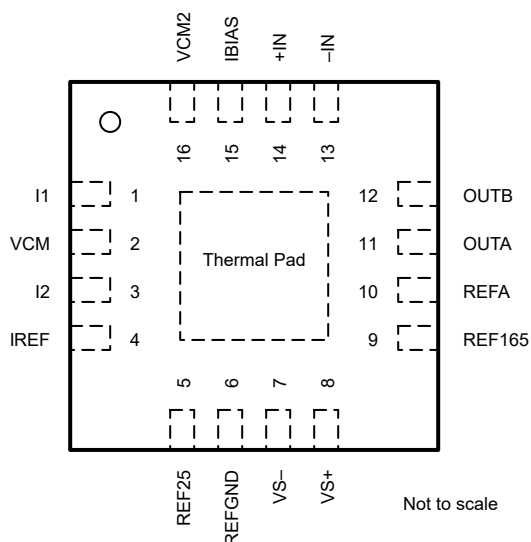
图 4-1. RGT 封装，16 引脚 VQFN (俯视图)
