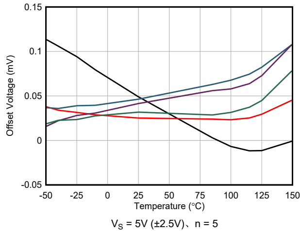
图 5-33. 辅助放大器偏移与温度间的关系
