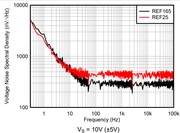
图 5-28. 电压基准噪声频谱密度
