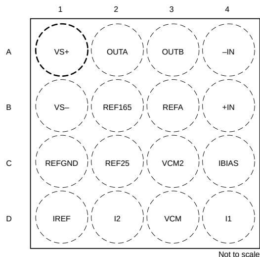
图 4-2. YBH 封装，16 引脚 DSBGA (俯视图)
