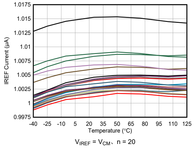
图 5-36. I_{REF} 与温度间的关系
