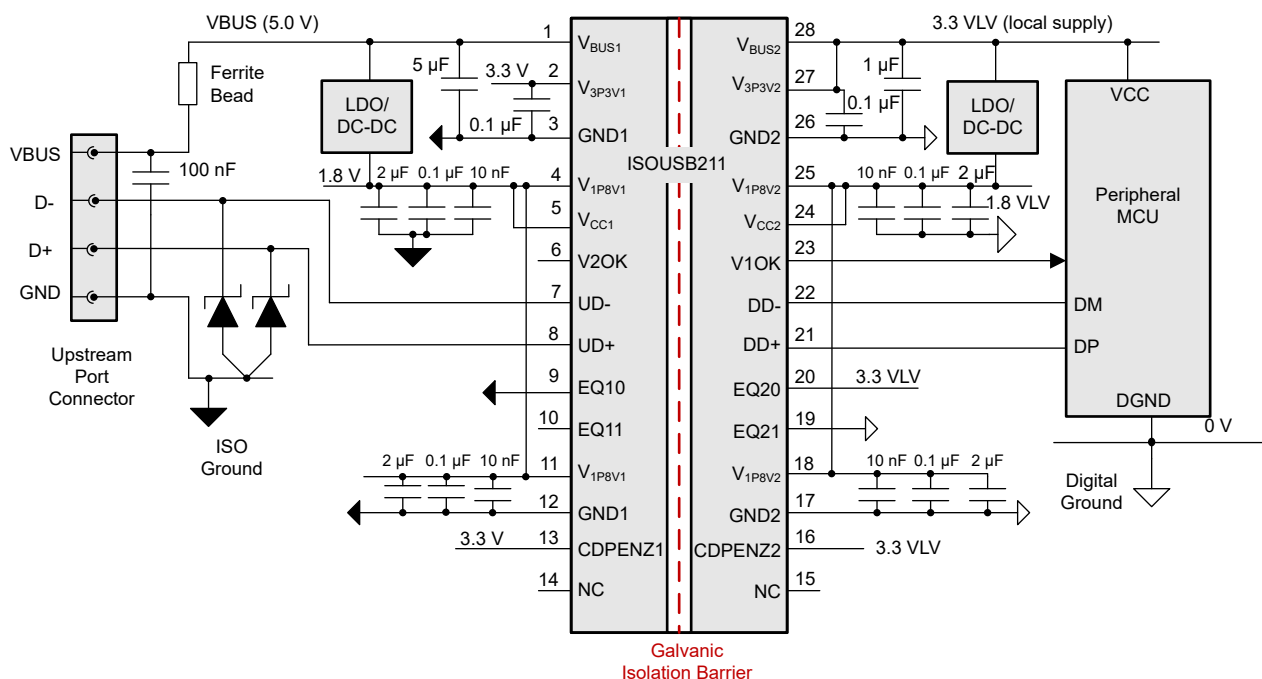
图 8-7. 将 ISOUSB211-Q1 与外部稳压器提供的 1.8V 电源搭配使用
