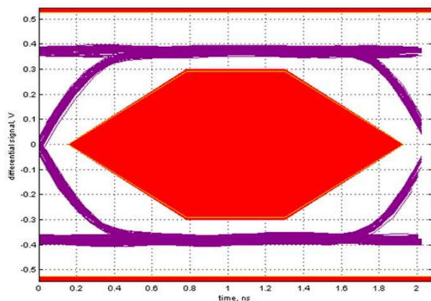
图 5-3. 通过 ISOUSB211-Q1 实现的典型高速 (480Mbps) 眼图
