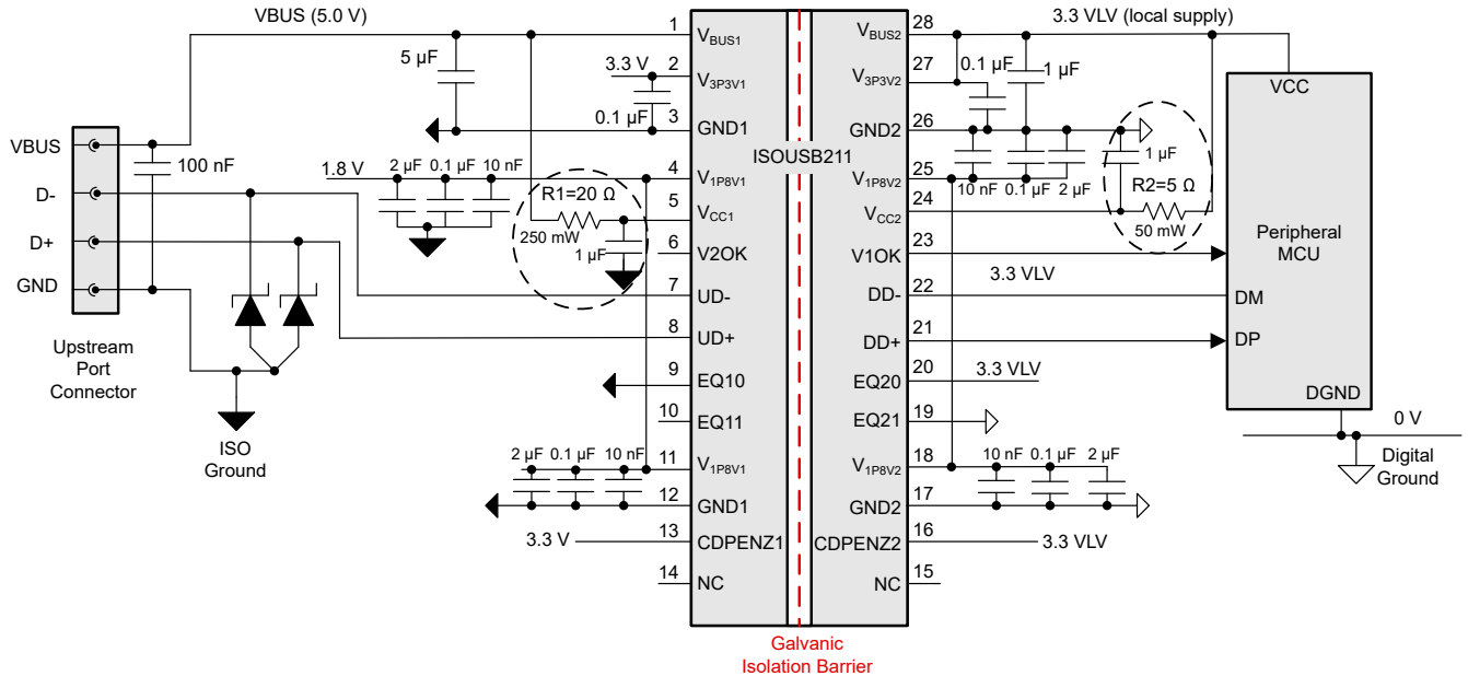
图 8-8. 将 ISOUSB211-Q1 与电阻器串联 V_{CCx} 引脚搭配使用
