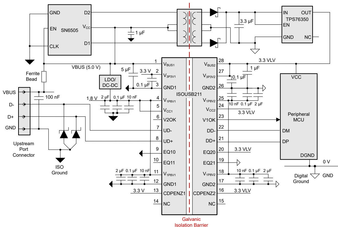
图 8-3. 采用 ISOUSB211-Q1 的隔离式总线供电外设
