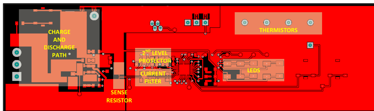
Figure 11-7. Top Layer
