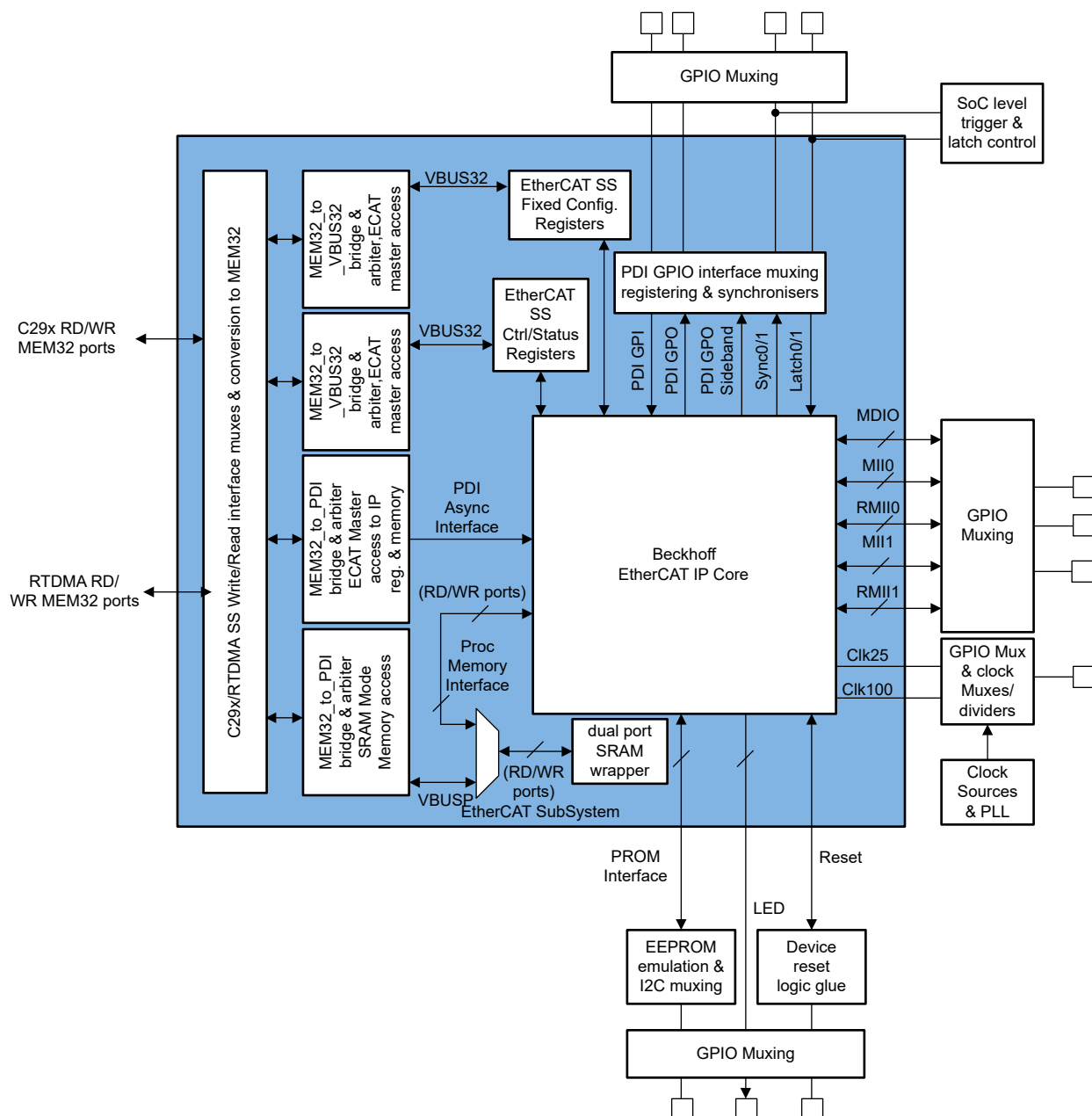
Figure 31-9. ESCSS Wrapper
