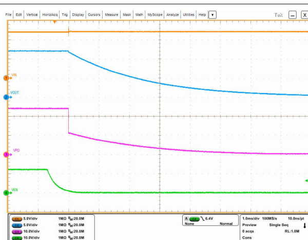
Figure 5-7. Disable Using EN
