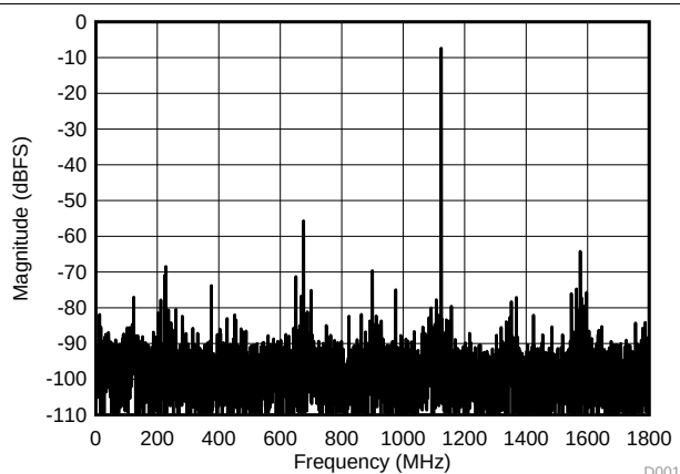
Figure 6-9. Spectrum DES Mode
