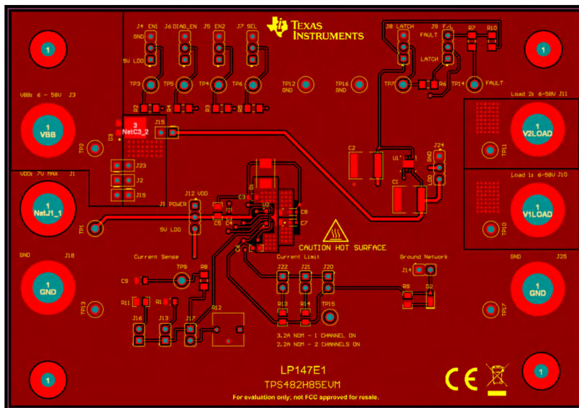
Figure 3-2. Top Layer
