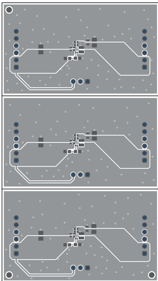
Figure 3-2. Top Layer
