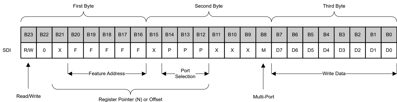
Figure 7-5. TXE8116-Q1 SPI SDI Data Frame Format
