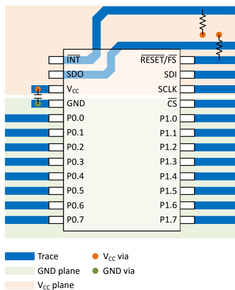
Figure 8-6. TXE8116-Q1 Layout
