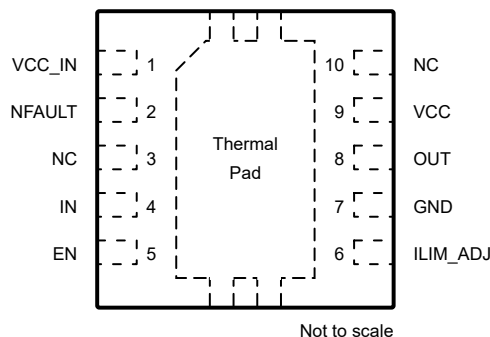
Figure 5-2. TIOS102 DRC, 10-Pin VSON (Top View)
