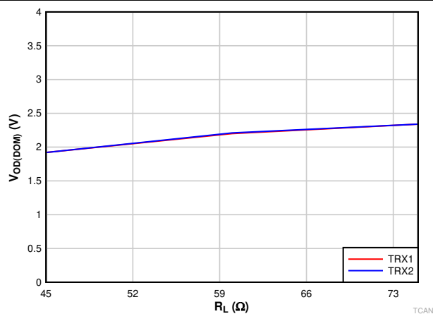
A. V_{CC} = 5\text{ V} Temp = 25°C
