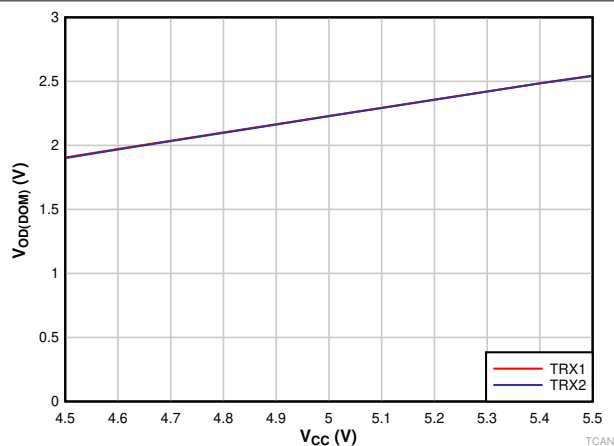
A. Temp = 25°C R_L = 60\ \Omega
