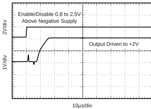
ENABLE ( 1\Omega Load)
