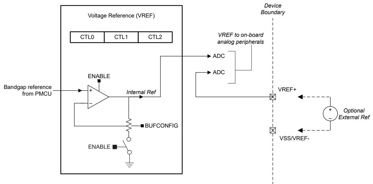
Figure 8-2. VREF module
