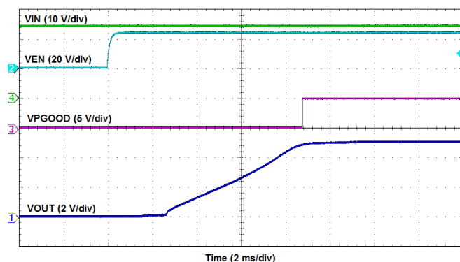
Figure 29. Enable Turn-ON
