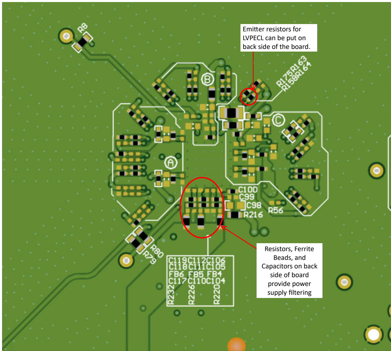
Figure 9-11. Bottom Layer
