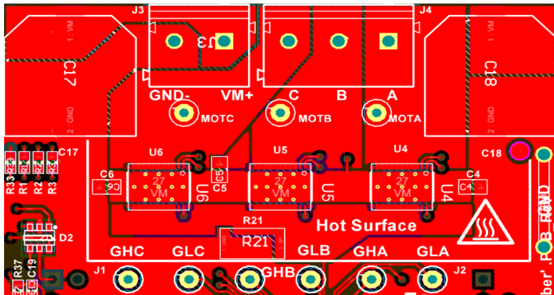
Figure 6-2. Top Layer
