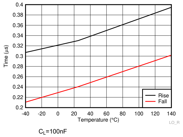
Figure 6-26. LO Rise andamp; Fall Time
