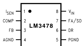
Figure 4-2. 8-Pin SOIC (D) Package (Top View)
