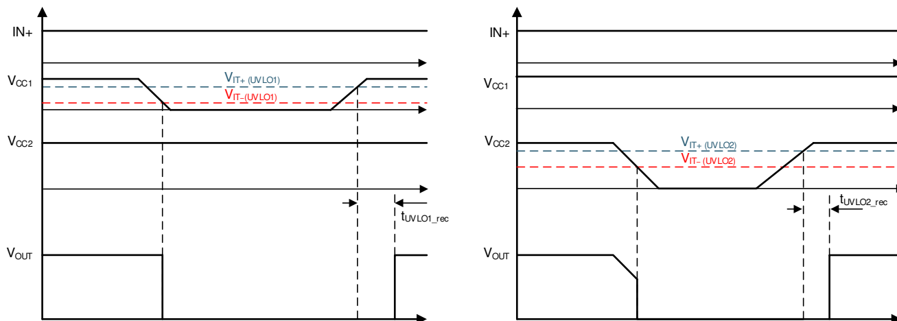
図 8-9. UVLO Functions
