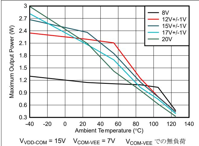
図 6-7. プリレギュレートされた入力電圧に対する SOA ディレーティング曲線
