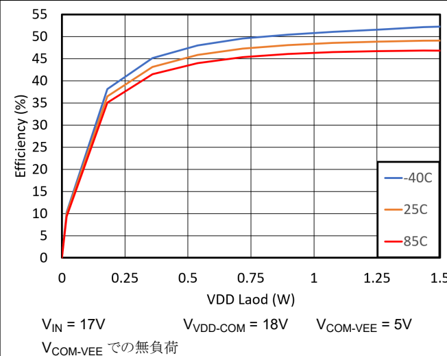
図 6-3. V_{VDD-COM} における効率と負荷との関係
