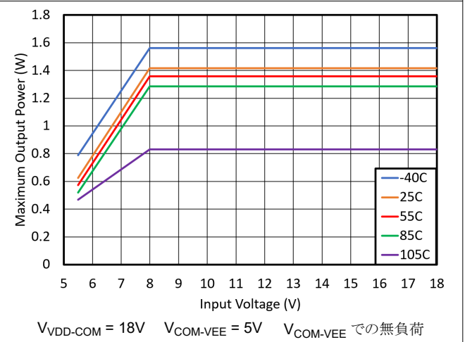
図 6-8. バッテリ直接接続を想定した入力電圧範囲が広い場合の SOA ディレーティング曲線
