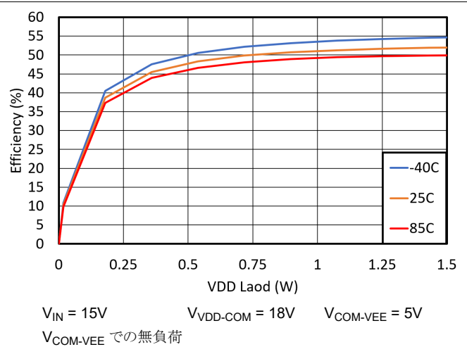
図 6-2. V_{VDD-COM} における効率と負荷との関係
