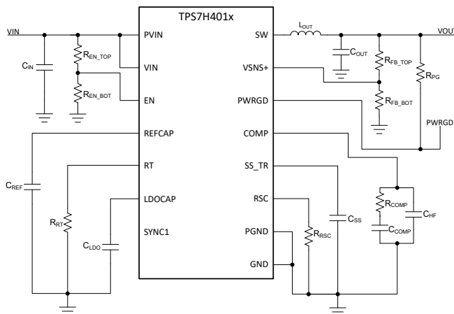
概略回路図
