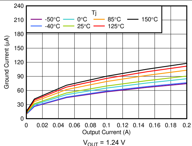
6-12. I_{\text{GND}} vs I_{\text{OUT}}
