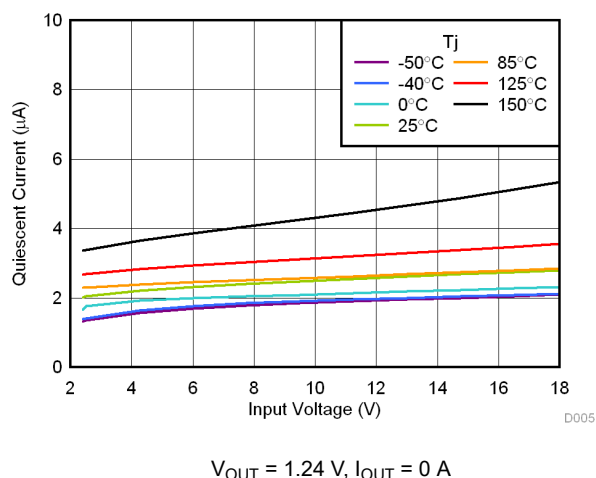
6-10. I_{\text{Q}} vs V_{\text{IN}}
