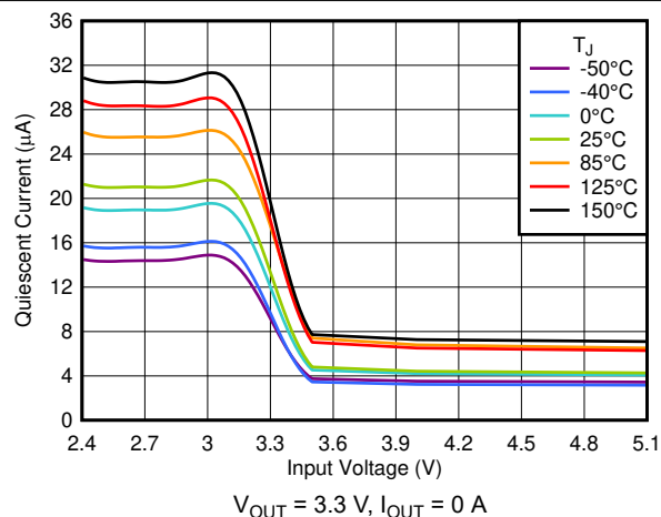
6-11. I_{\text{Q}} vs V_{\text{IN}}
