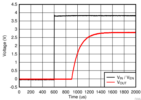
図 7-5. Start-Up
