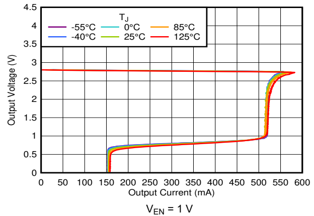
図 5-44. Current Limit
