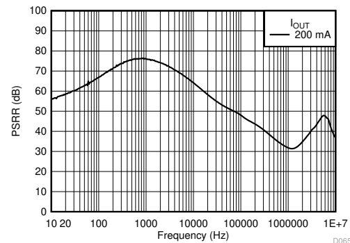
図 7-6. PSRR
