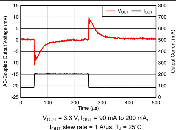
FIG 6-62. Load Transient
