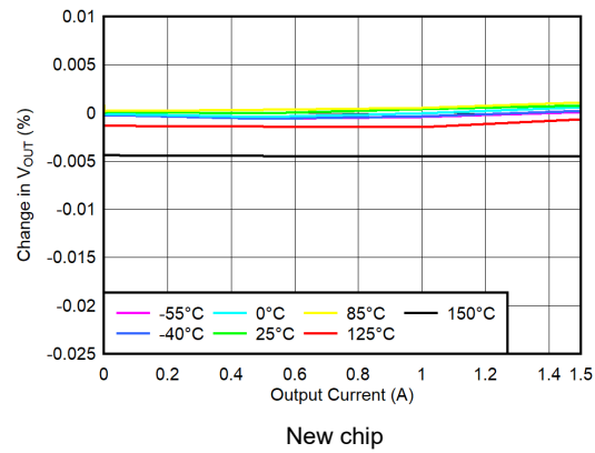
图 5-4. Load Regulation
