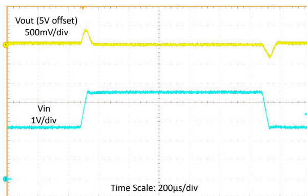
図 8-5. シャットダウン波形
