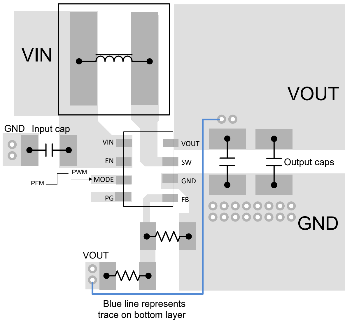
図 8-12. レイアウト例
