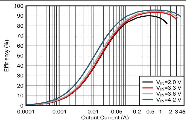
図 6-1. 効率と出力電流との関係 ( V_{OUT} = 5V )
