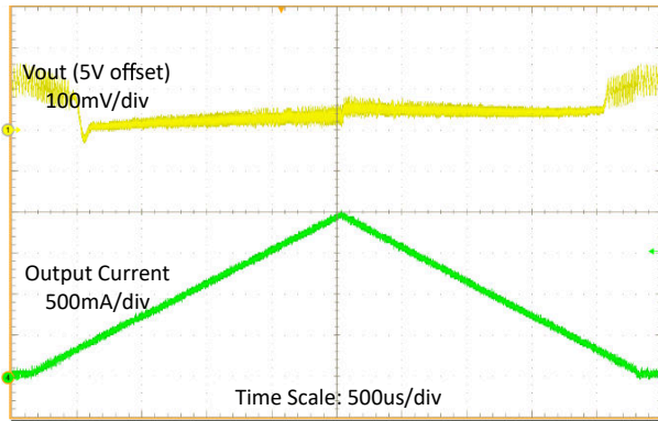
図 8-8. 負荷スイープ
