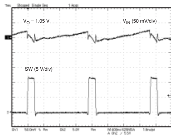
図 12. 入力電圧リップル ( I_O = 2A )
