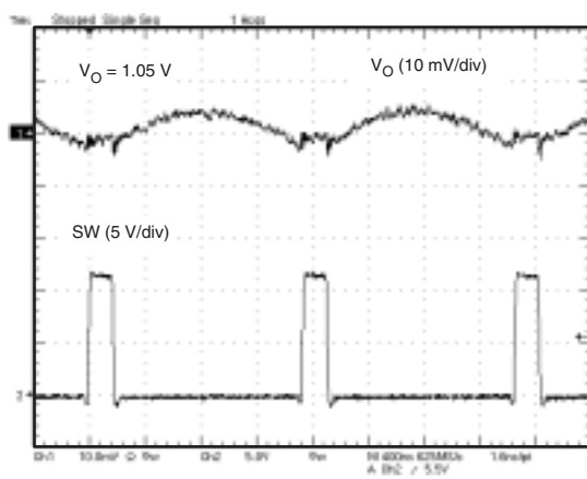
図 11. 出力電圧リップル ( I_O = 2A )
