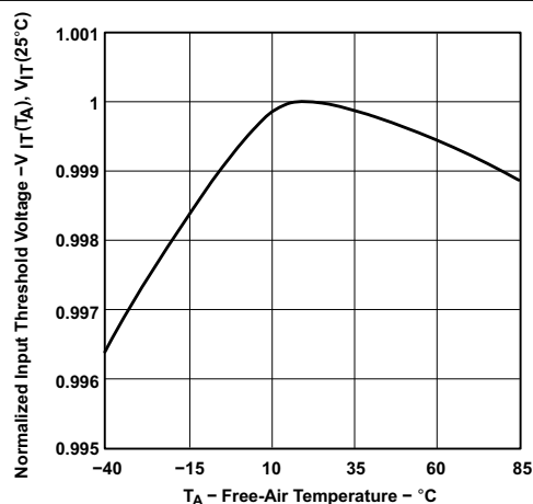
図 6-2. 正規化された入力スレッシュホールド電圧と V_{DD} での自由通気温度との関係
