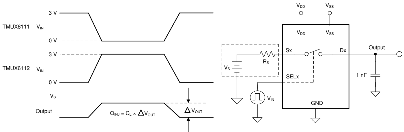
図 8-6. 電荷注入測定時の設定
