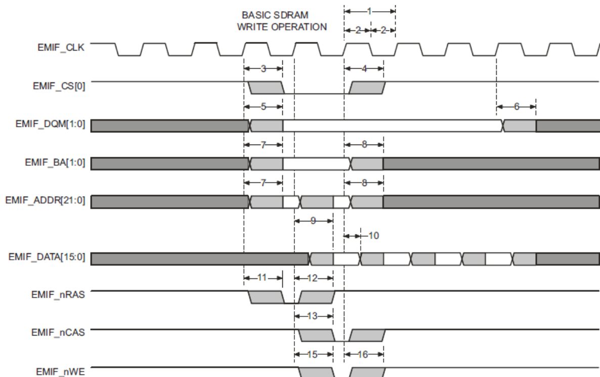
図 4-16 基本 SDRAM ライト動作
