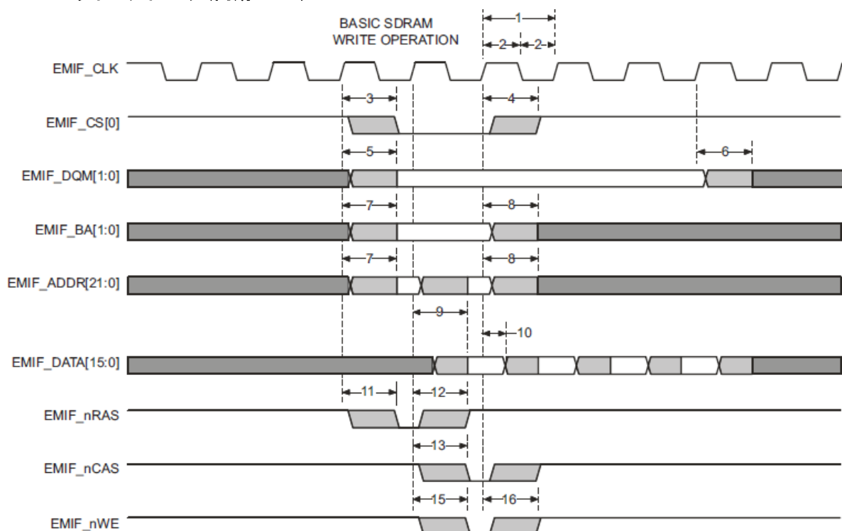
図 4-16 基本 SDRAM ライト動作
