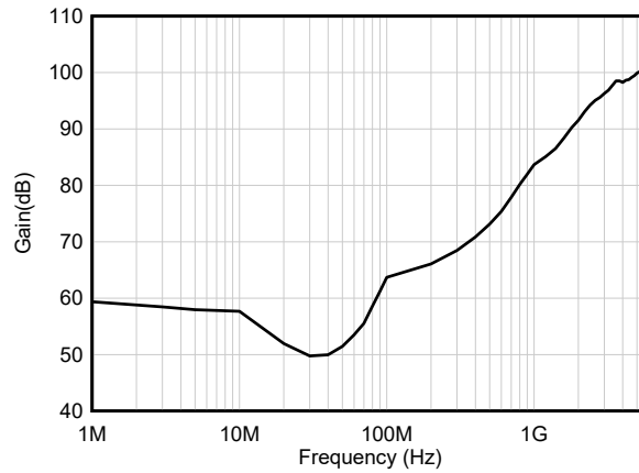
図 5-41. 入力における EMIRR (電磁干渉除去比) と周波数との関係
