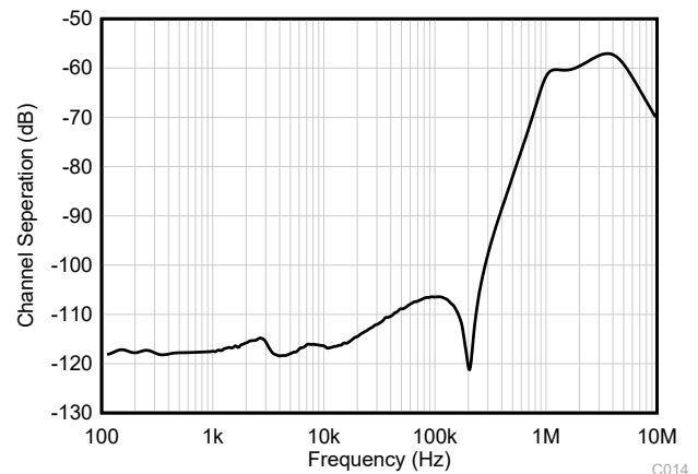
図 5-40. チャネル分離と周波数との関係
