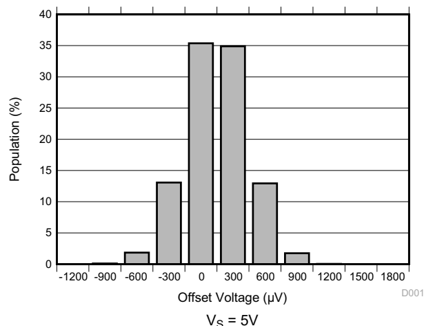
図 7-1. オフセット電圧の分布ヒストグラム
