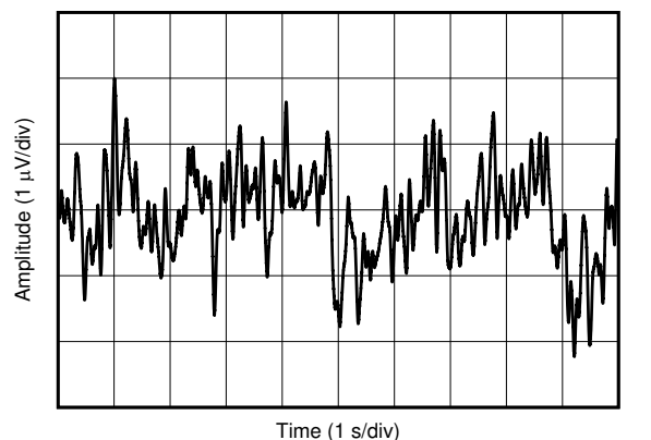
図 7-17. 0.1Hz~10Hz の統合電圧ノイズ
