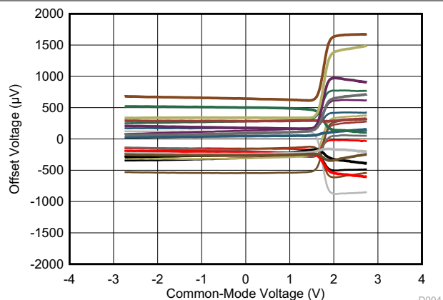
図 7-4. オフセット電圧と同相との関係
