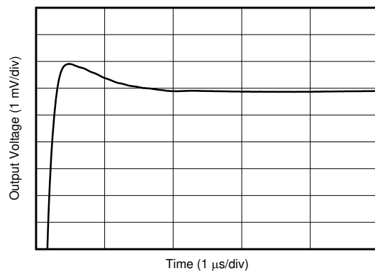
図 7-32. 大信号のセトリング・タイム (正)
