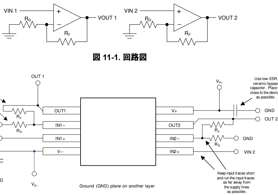
図 11-2. レイアウト例
