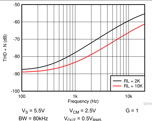
図 7-19. THD+N と周波数との関係
