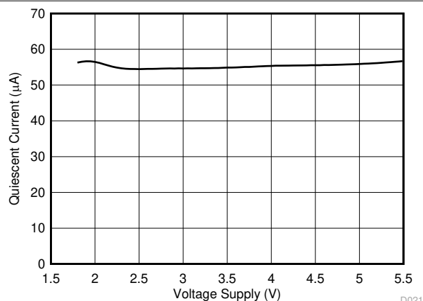
図 7-21. 静止電流と電源電圧との関係
