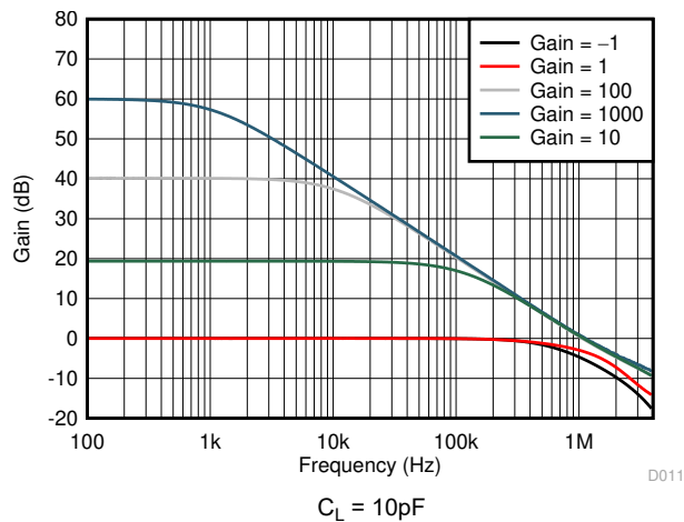
図 7-11. 開ループのゲインと周波数との関係
