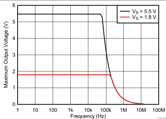
図 7-34. 最大出力電圧と周波数との関係
