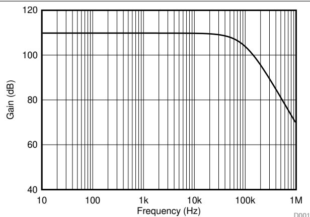
図 9-4. フォトダイオード・アンプ回路の AC ゲイン結果
