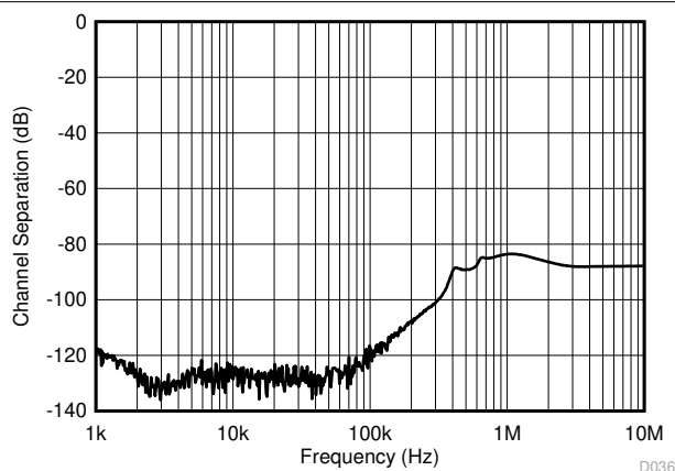
図 7-36. チャネル・セパレーション
