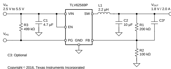
概略回路図
