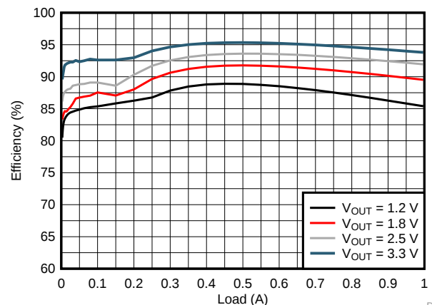
5V入力電圧時の効率
