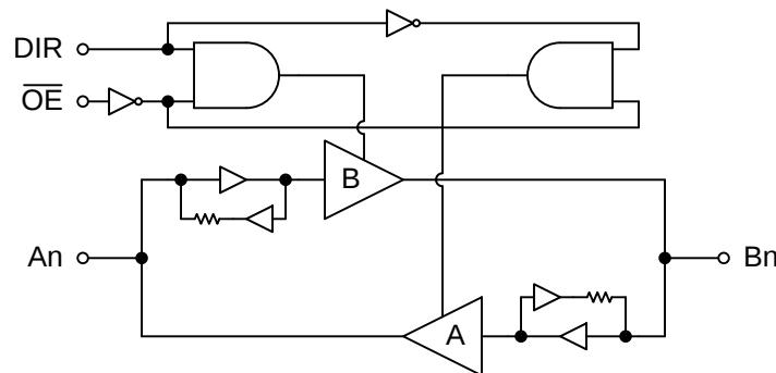
概略回路図
