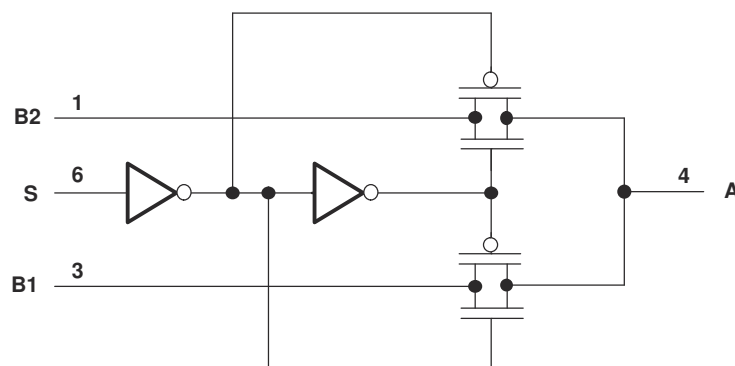
図 7-1. 論理図 (正論理)
