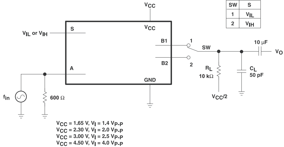
図 6-9. 全高調波歪
