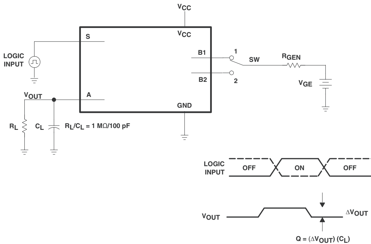
図 6-8. チャージインジェクション試験
