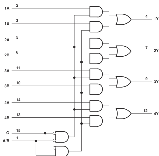
論理図 (正論理)
