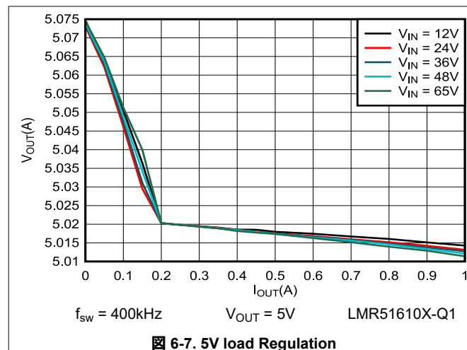
図 6-7. 5V load Regulation
