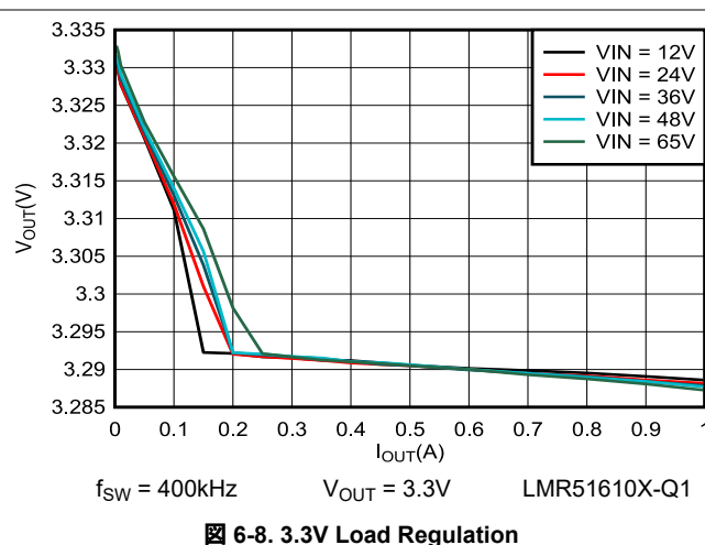
図 6-8. 3.3V Load Regulation
