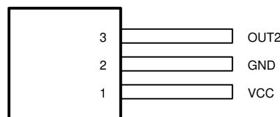
図 5-6. DU、FD バージョンの LPG パッケージ 3 ピン TO-92 上面図
