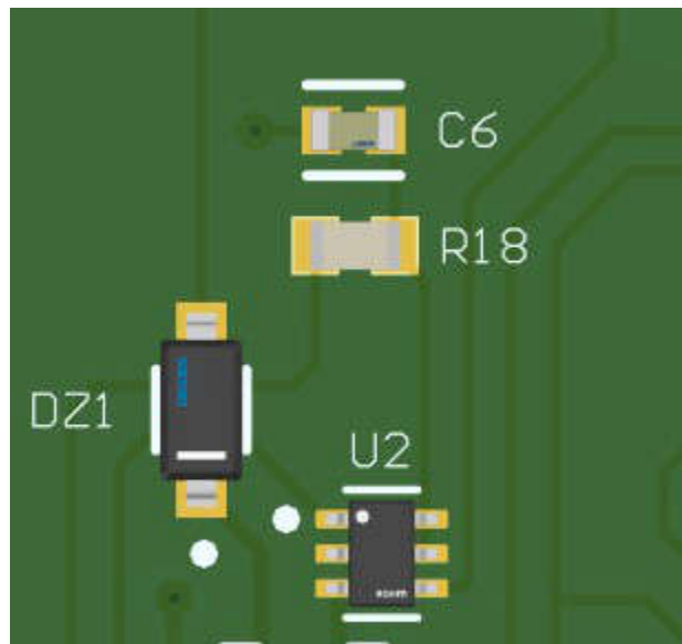
图 2-2. GPI 保护块
