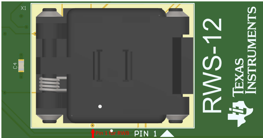
图 3-8. RWS/RWB 插座
