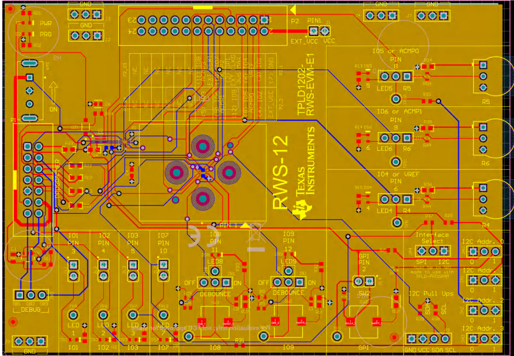
图 4-3. TPLD1202-RWS-EVM 布局
