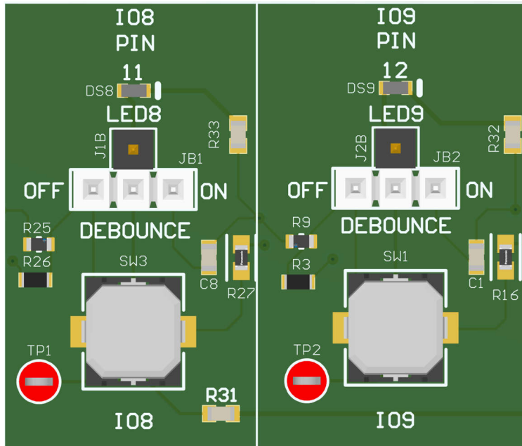
图 2-6. 开关/LED 块
