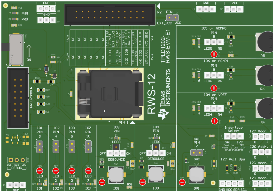
图 4-4. TPLD1202-RWS-EVM 电路板正面
