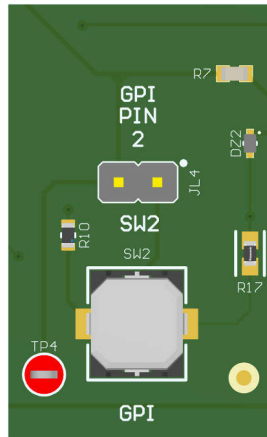
图 2-7. 开关模块
