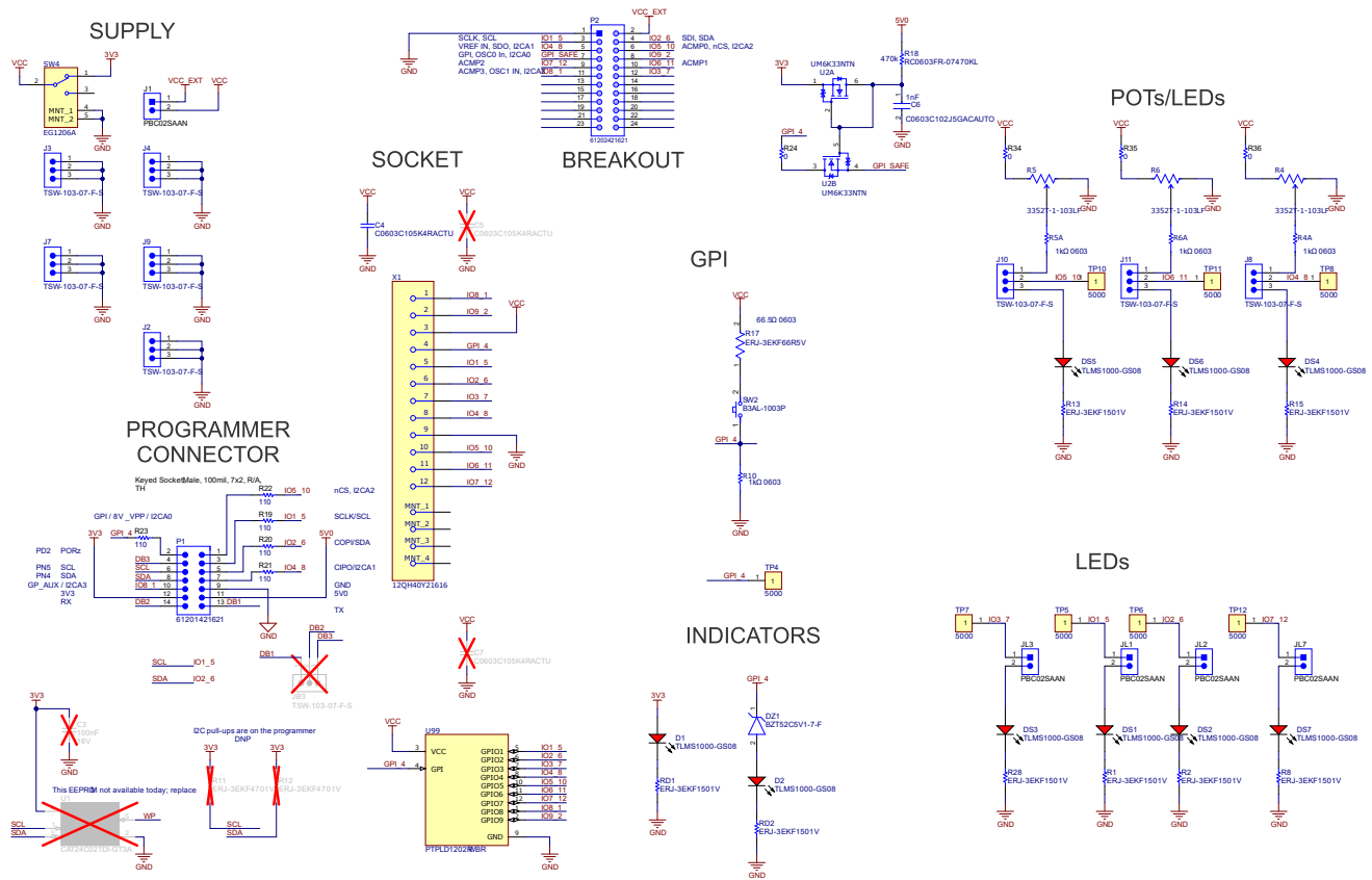
图 4-1. TPLD1202-RWS-EVM 原理图 1
