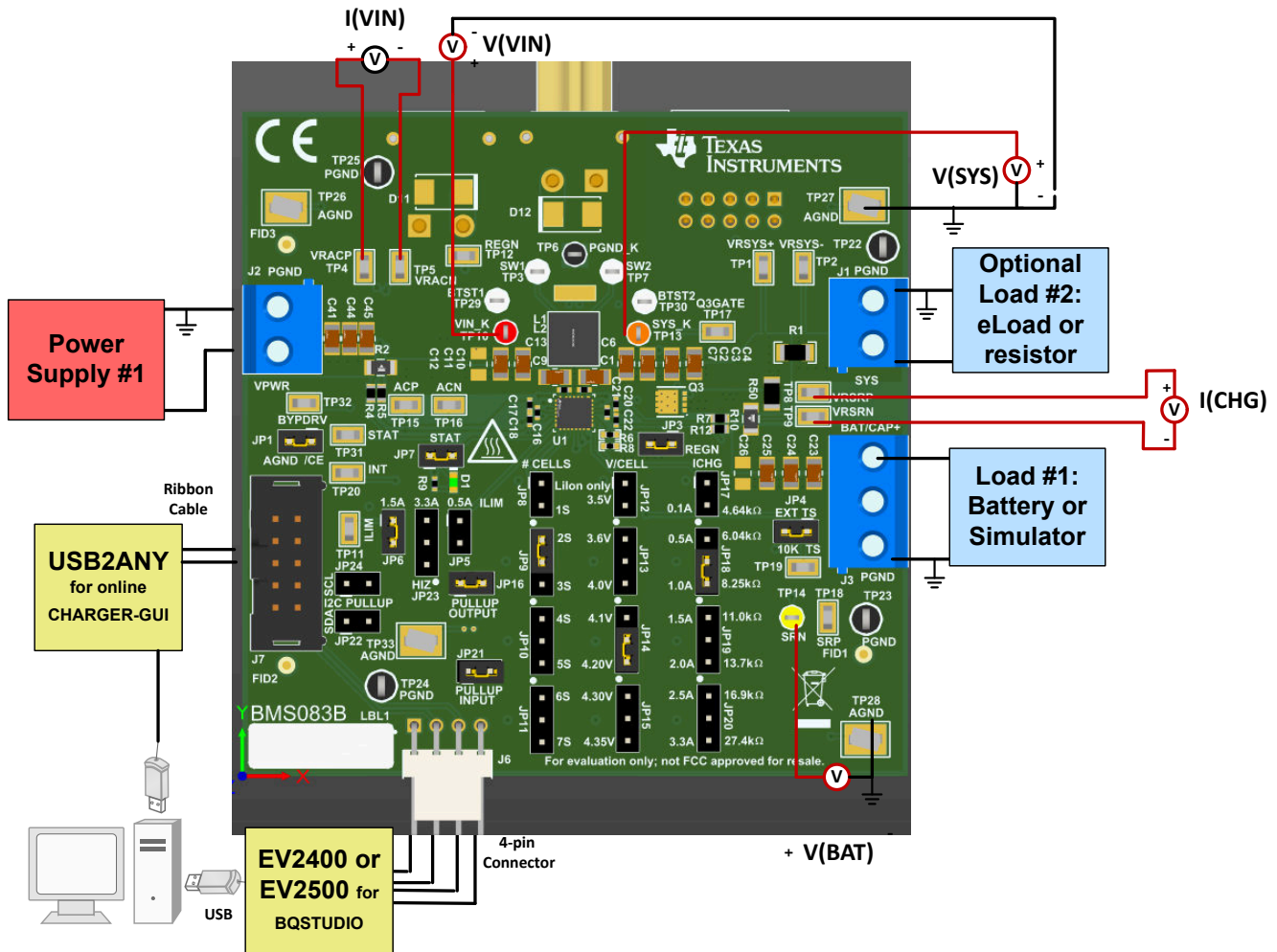
图 2-1. BQ25690EVM 的测试设置
