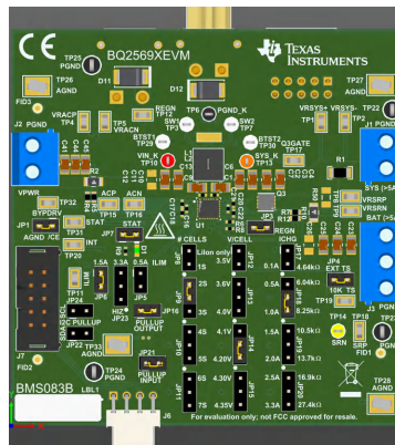
BQ25690EVM REV B 硬件电路板
