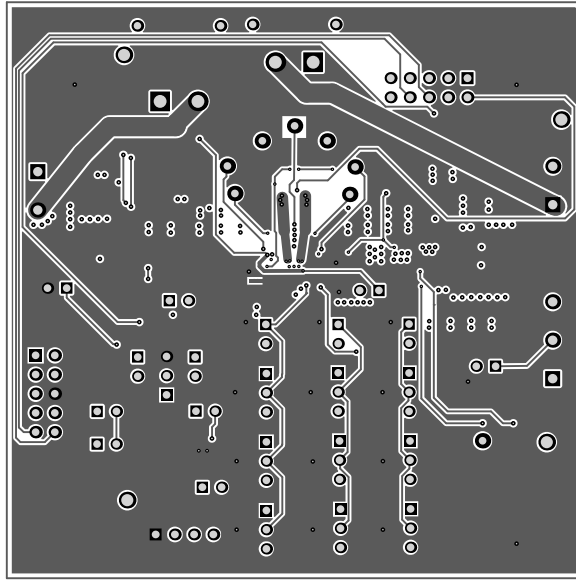
图 4-5. BMS083B 内部 2 层
