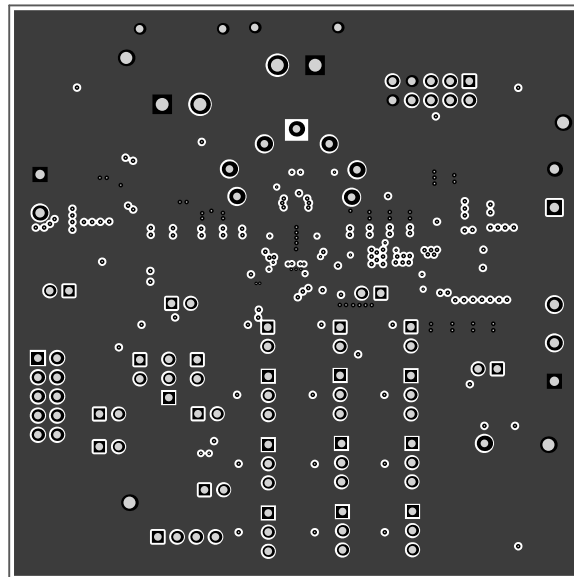
图 4-4. BMS083B 内部 1 层
