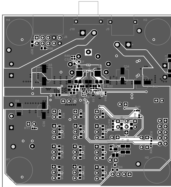
图 4-6. BMS083B 底视图
