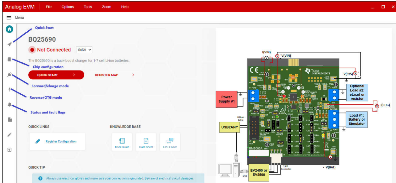
图 3-5. BQ25690EVM 主页
