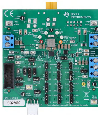
BQ2569X/9X-Q1EVM 硬件板
